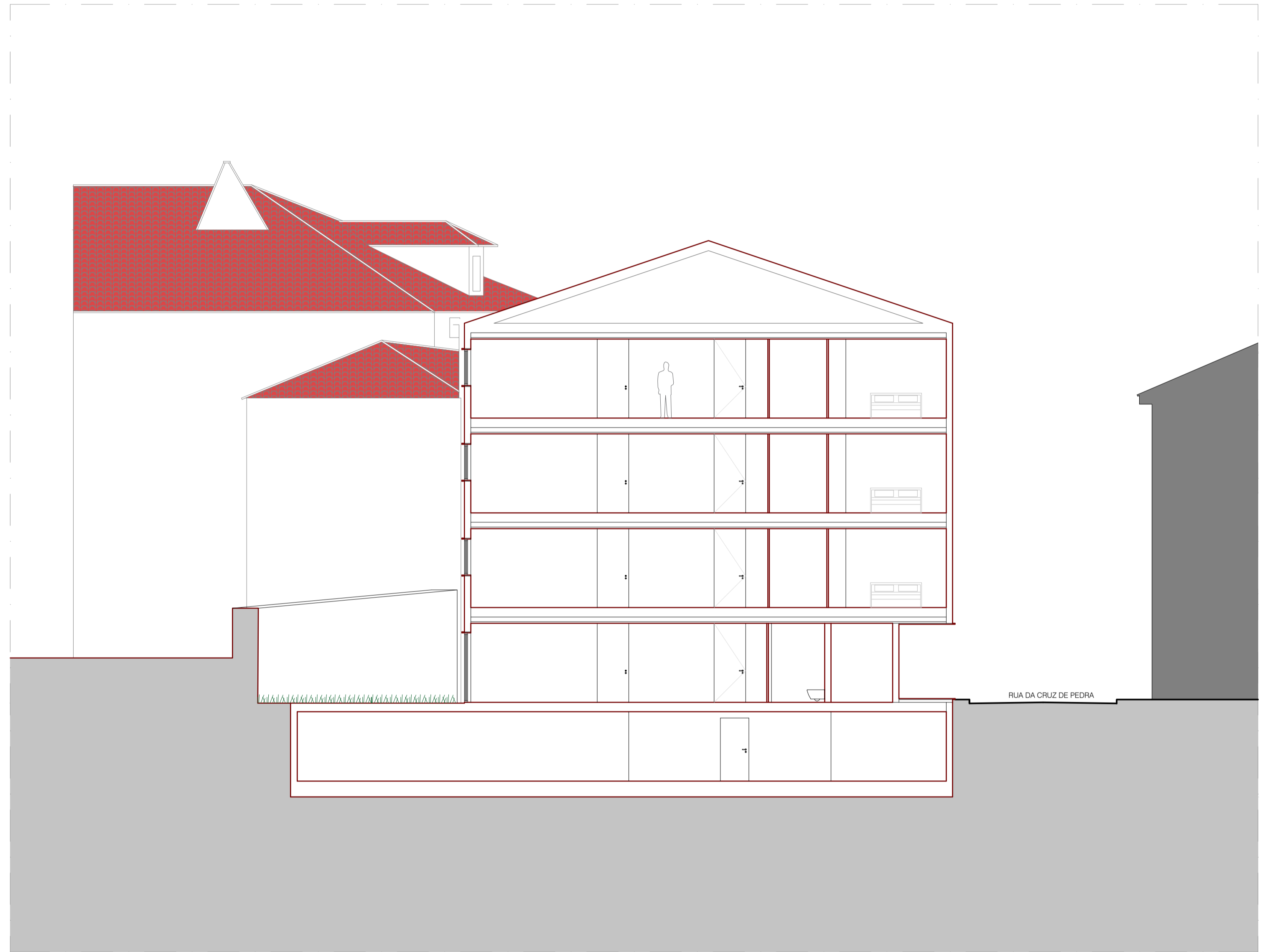
02 - CORTE B PROPOSTA escala 1:100
