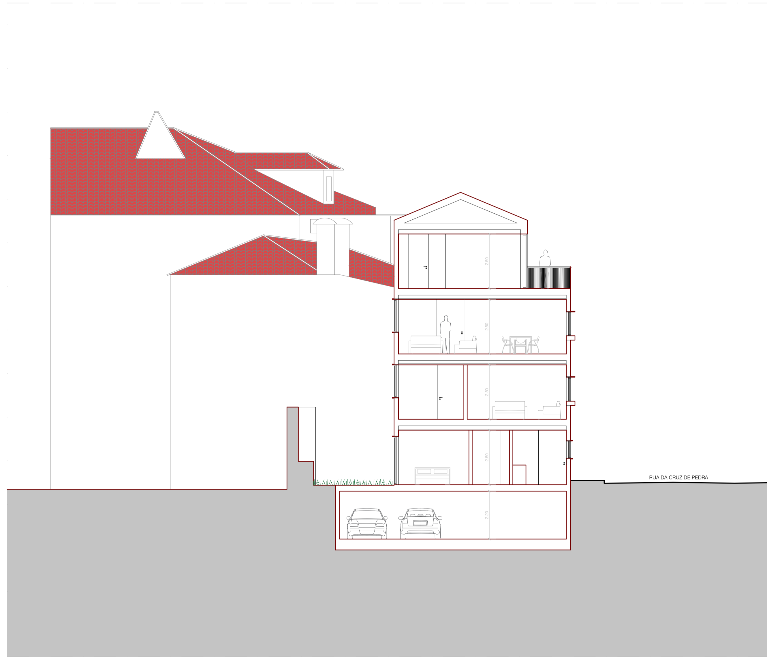
01 - CORTE A PROPOSTA escala 1:100
