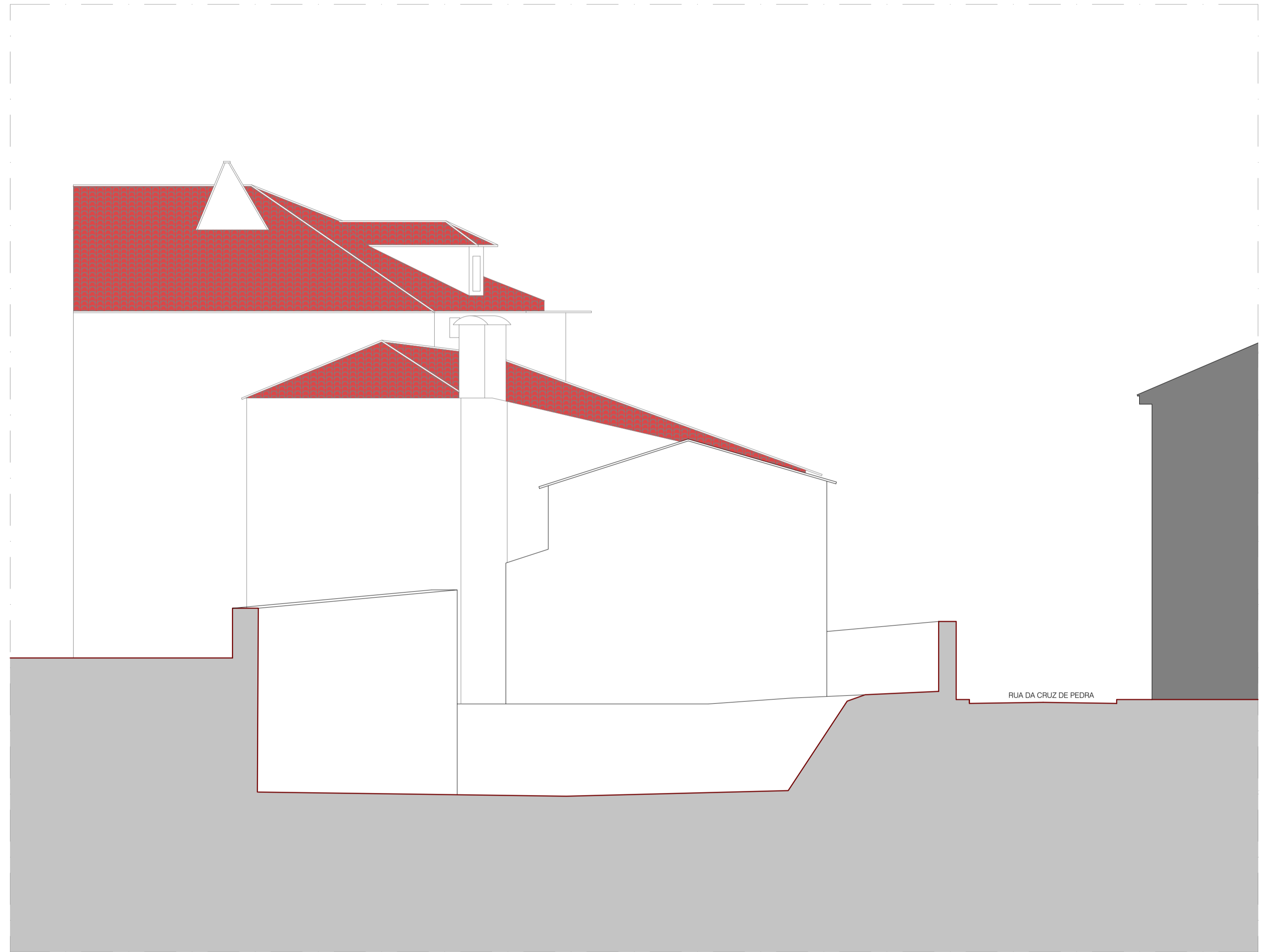
02 - CORTE B EXISTENTE escala 1:100
