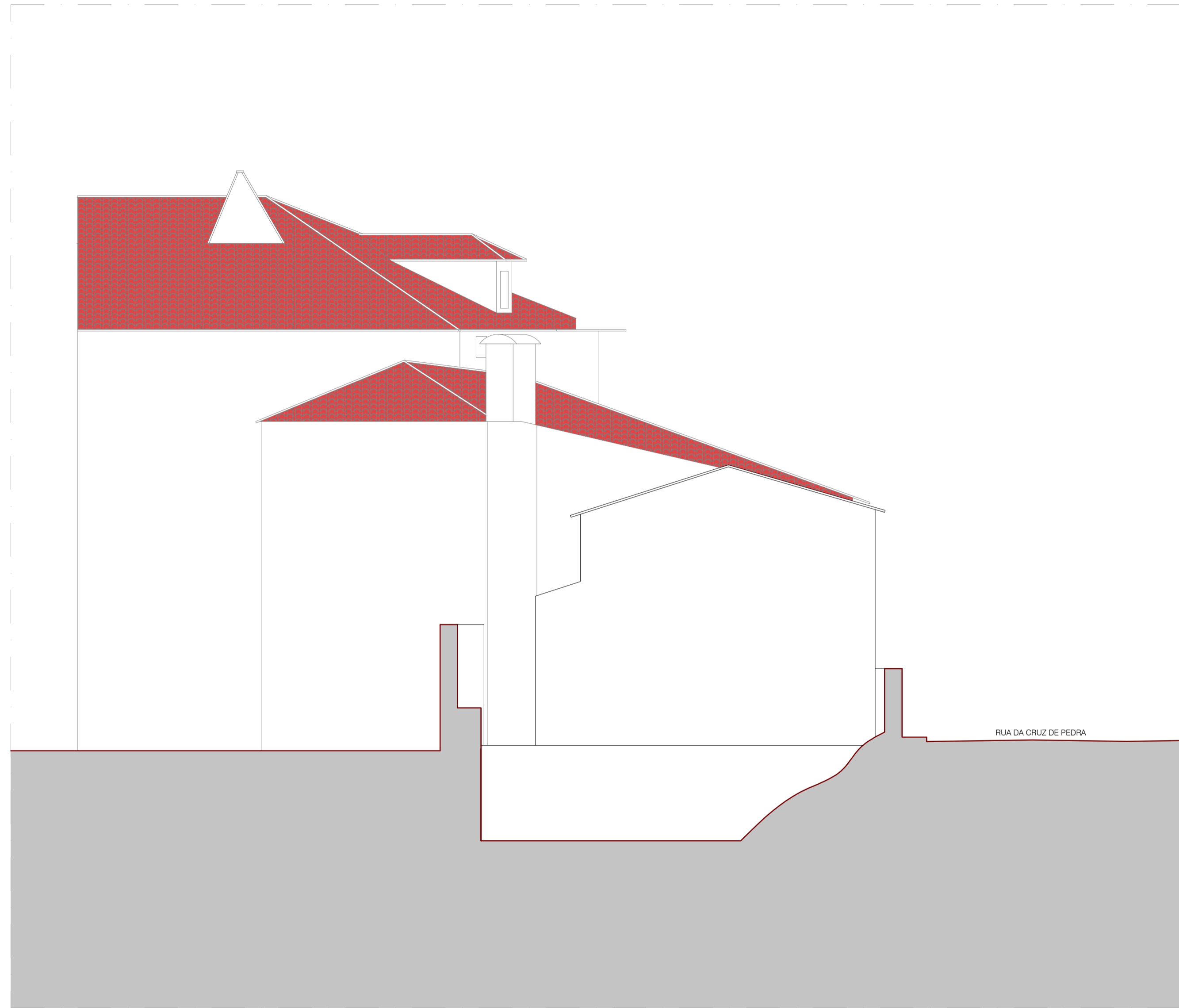
01 - CORTE A EXISTENTE escala 1:100
